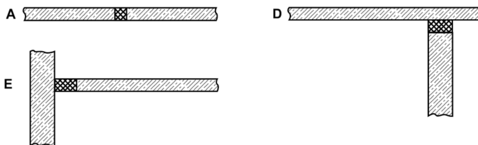
A: Decke - Decke / horizontal D: Decke - Wand / horizontal E: Wand - Decke / horizontal
